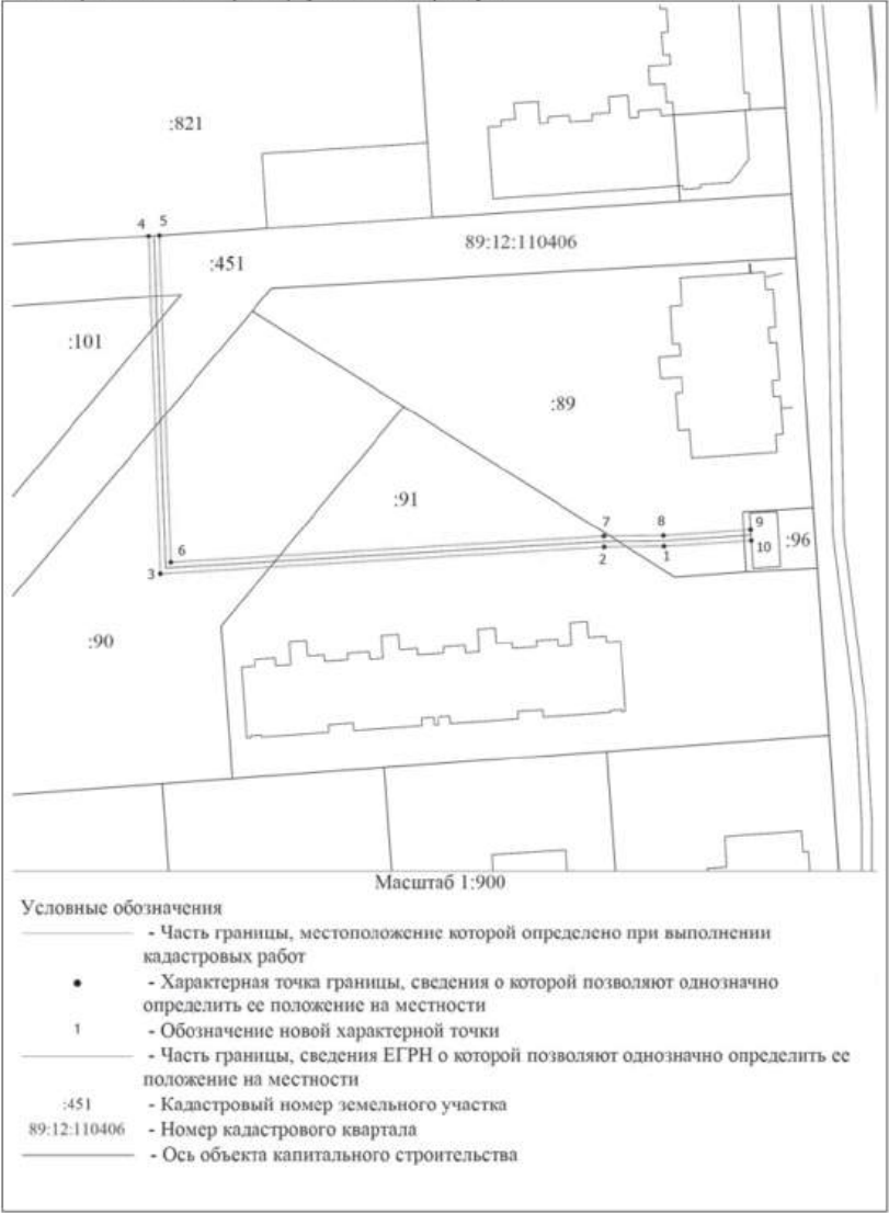
Раздел 4. Схема расположения границ публичного сервитута
